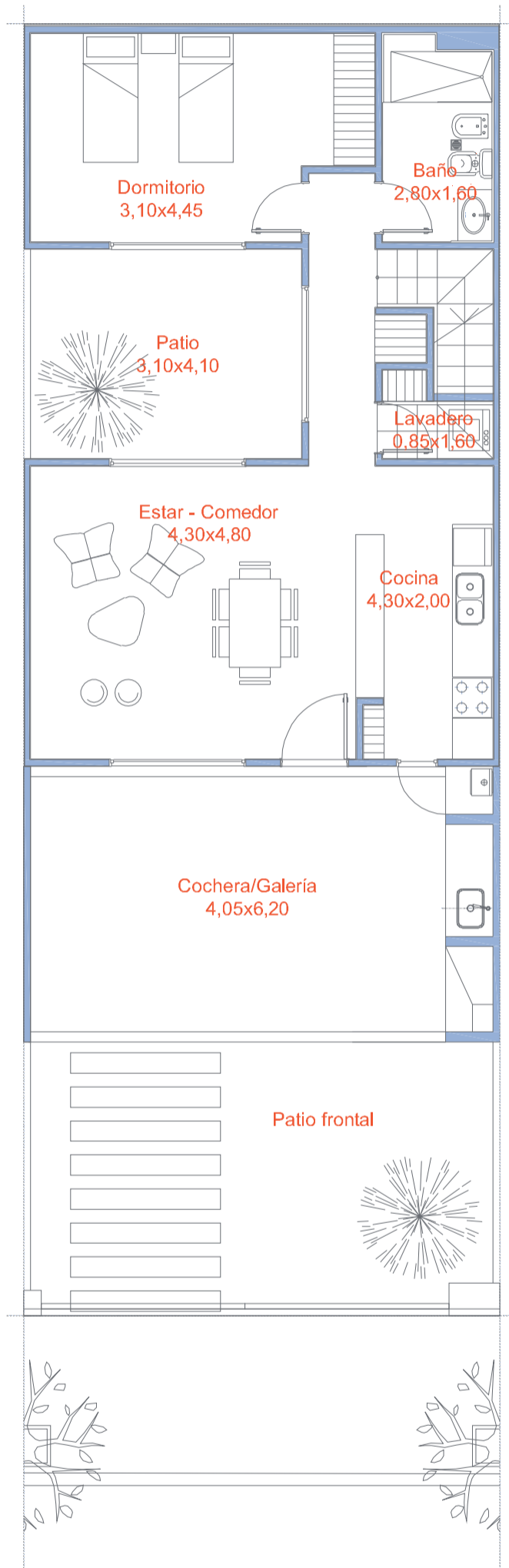
Planta baja
