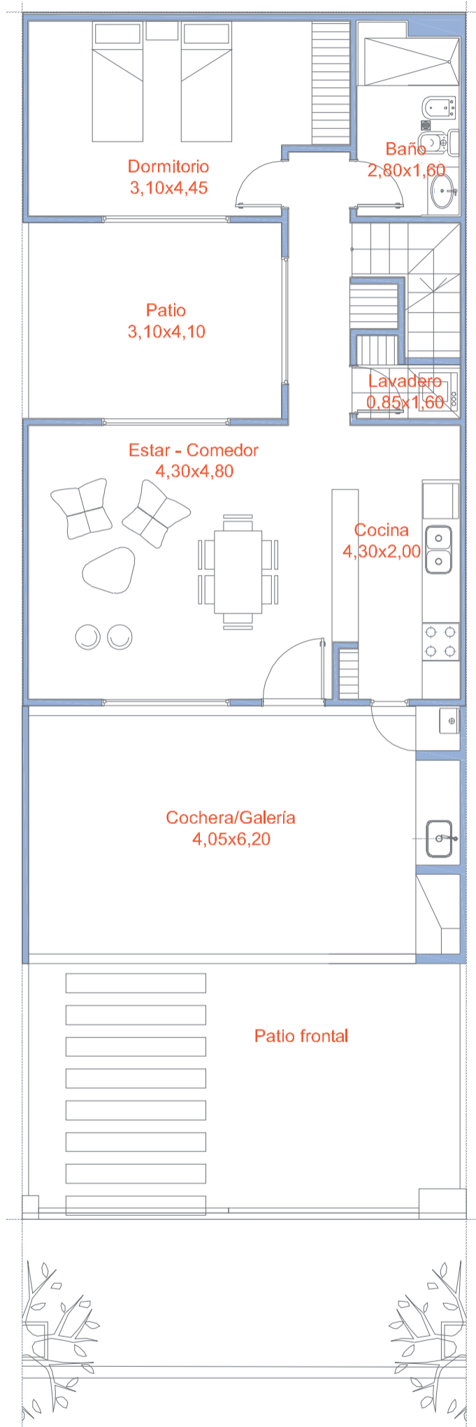
Planta baja
