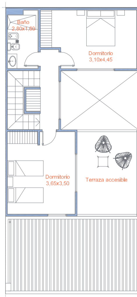
Planta alta
