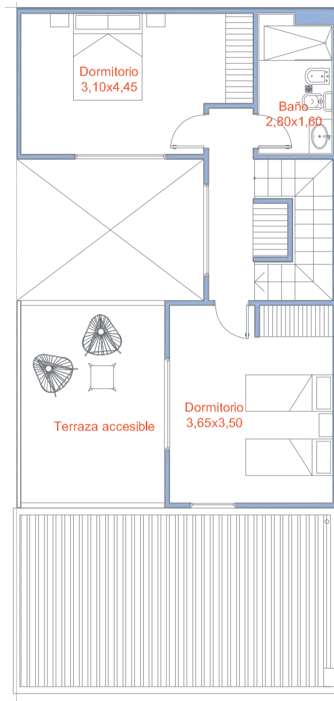
Planta alta
