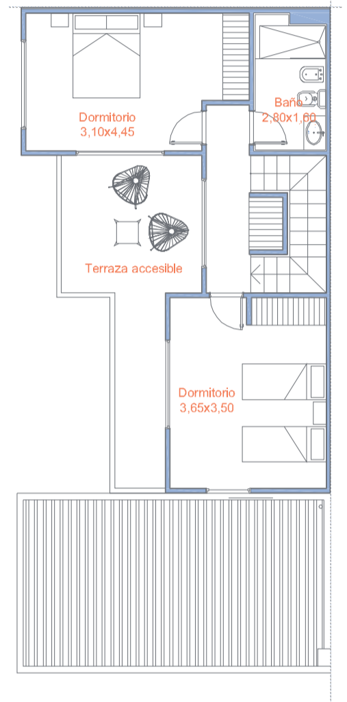
Planta alta
